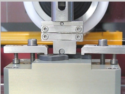
Zylinderrolle / Platte
