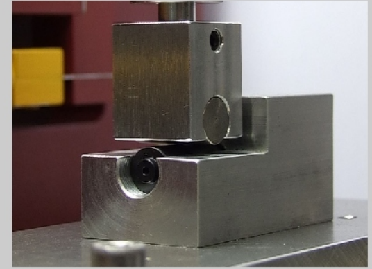
gekreuzte Zylinder
