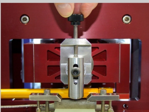
Niederhalter
