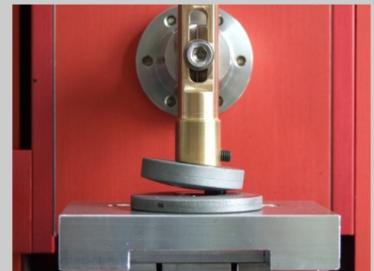
Kalotte / Platte
